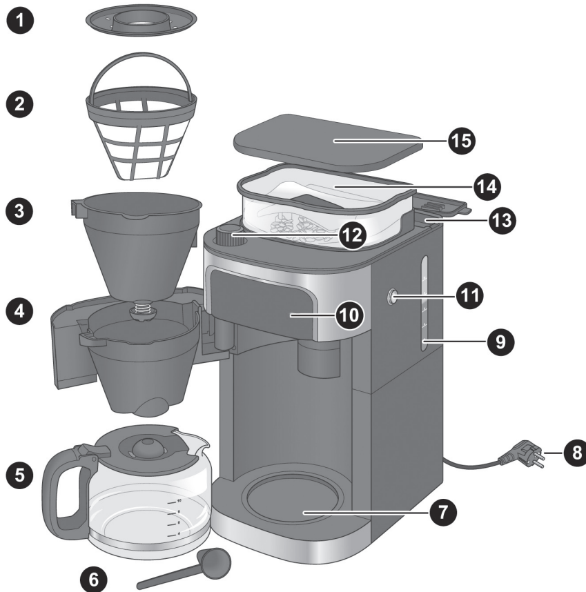
Fig. 1: Parti dell'apparecchio
