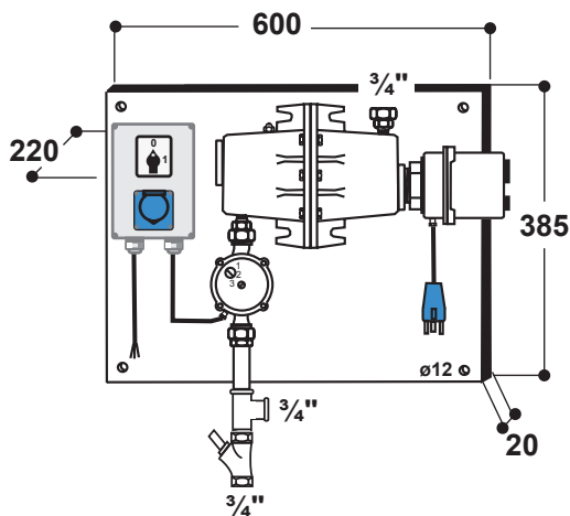
Abmaße • Dimensions • Габариты Mod. 303 / Mod. 300
