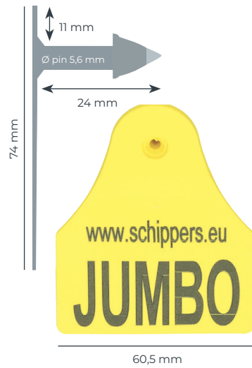
MS Tag Jumbo (Robust pin)
