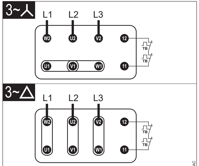
Afbeelding 4: 3~ STER / DRIEHOEK met optionele thermische detectoren (thermostaten)
