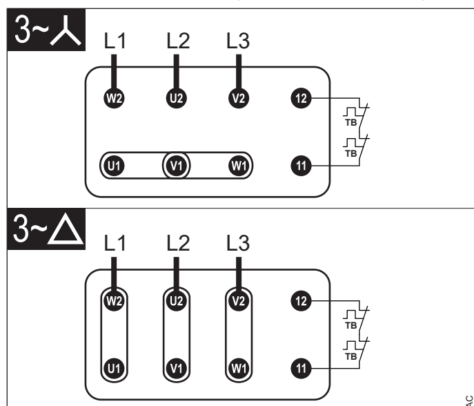
Ilustración 4: 3~ ESTRELLA / DELTA con detectores térmicos opcionales (termostatos)
