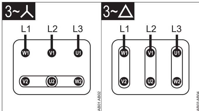
Afbeelding 3: 3~ STER / DRIEHOEK (standaard klemmenbord)
