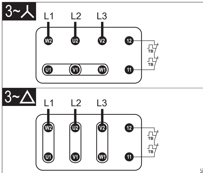
Fig. 4: 3~ ETOILE / TRIANGLE avec des détecteurs thermiques facultatifs (thermostats)
