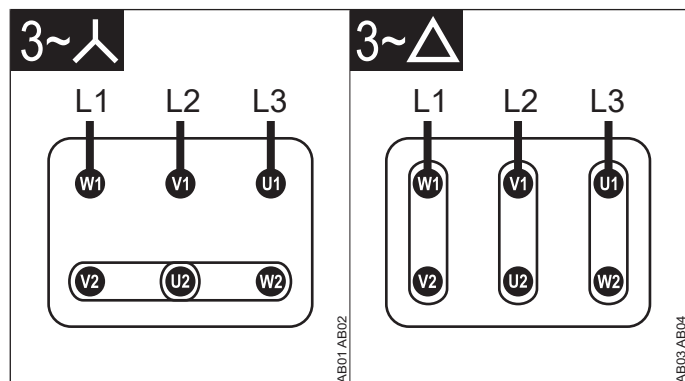
Abb. 3: 3~ STERN / DREIECK (Standard-Klemmenblock)
