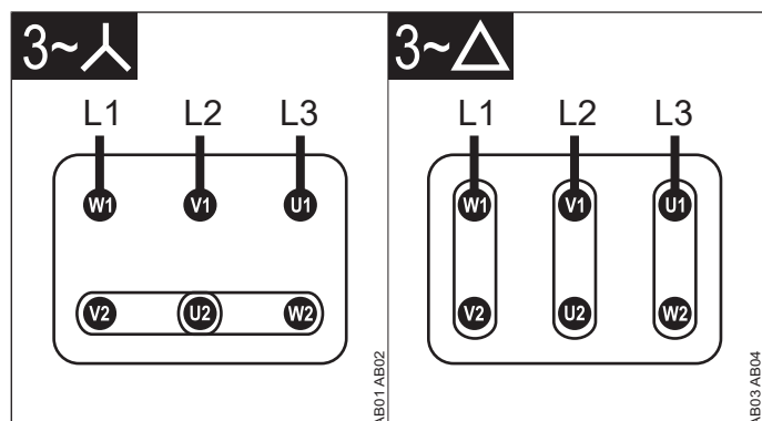
Ilustración 3: 3~ ESTRELLA / DELTA (bloque de terminales estándar)
