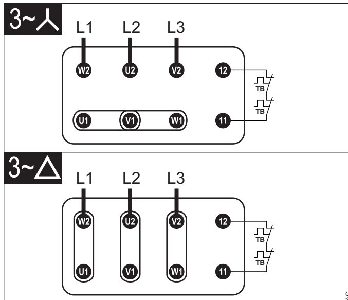
Abb. 4: 3~ STERN / DREIECK mit optionalen thermischen Detektoren (Thermostaten)
