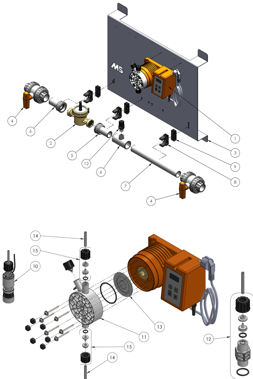
Abb. 1.1 Explosionszeichnung
