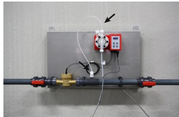
Abbildung 4: Druckluftschlauch anschließen
