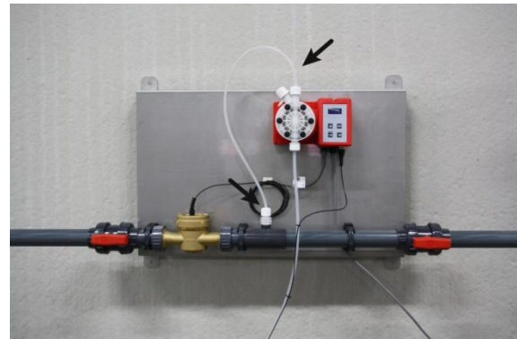
III. 4: Raccorder le tuyau de sortie
