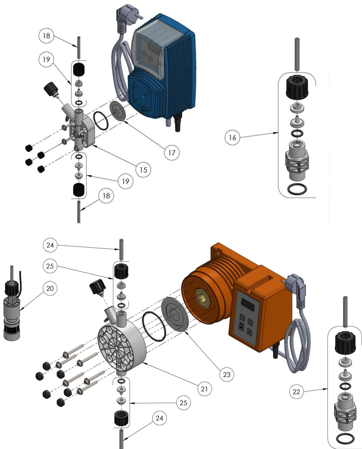
Fig 1.1 Vue en éclaté
