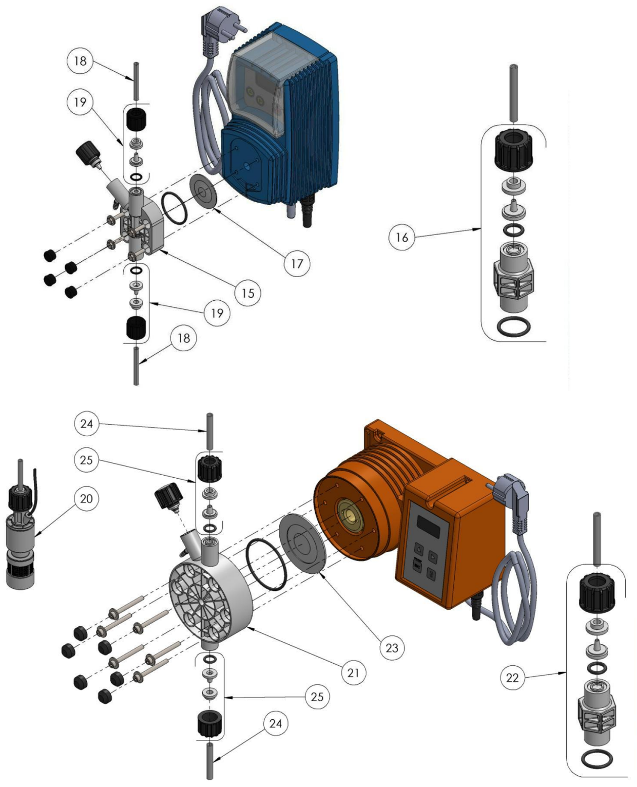
Abb. 1.1 Explosionszeichnung
