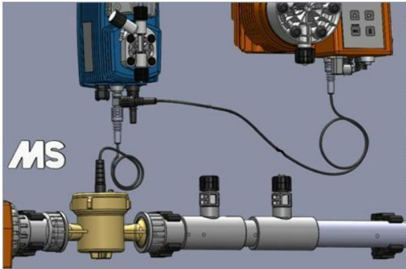
Abbildung 5: Anschließen Wasserzähler
