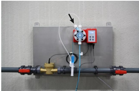
Imagen 15: Purgar el aire de la bomba
