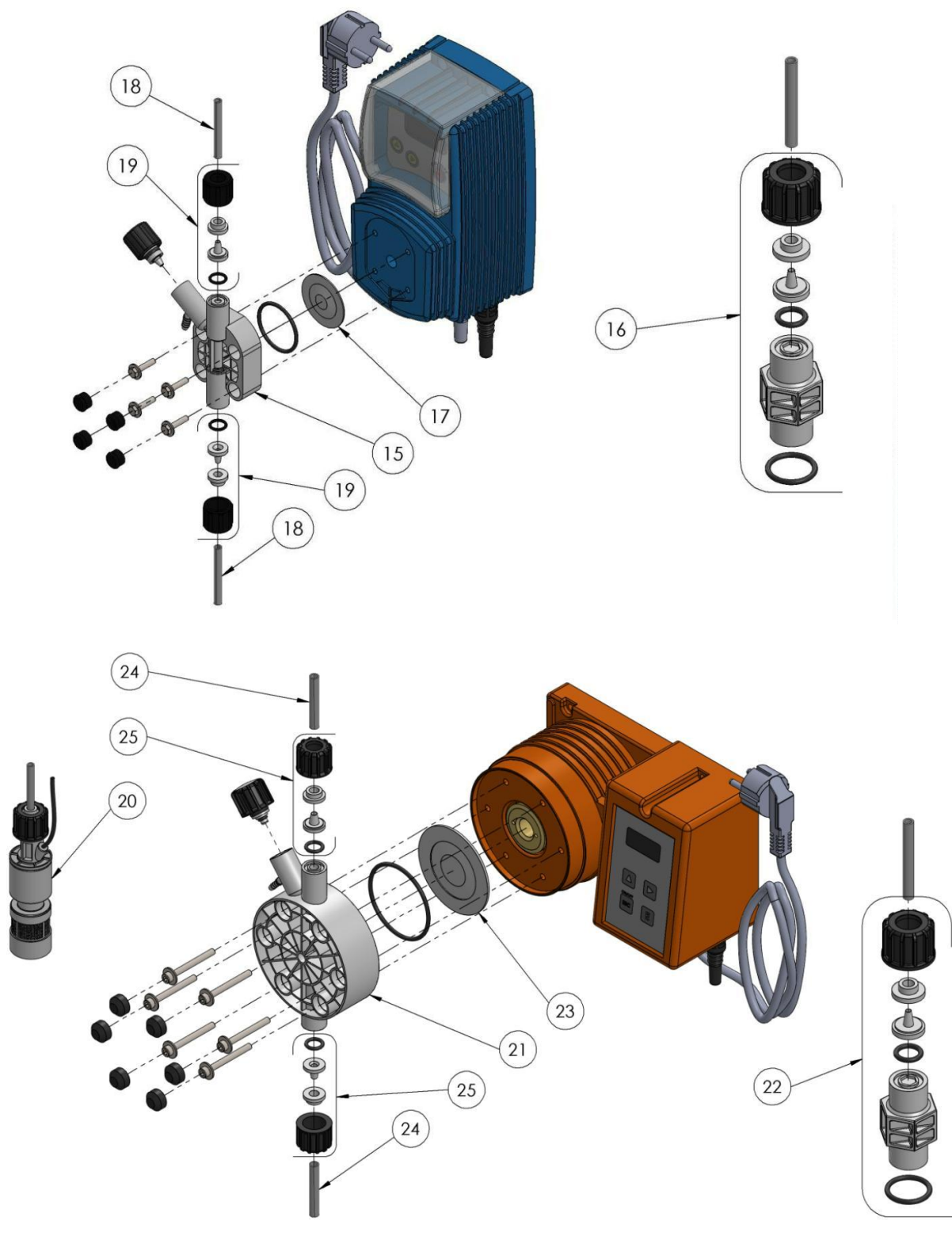
Fig 1.1 Vue en éclaté
