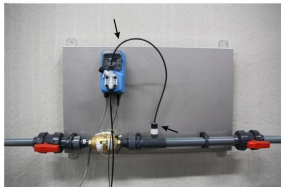
II. 4: Raccorder le tuyau de sortie
