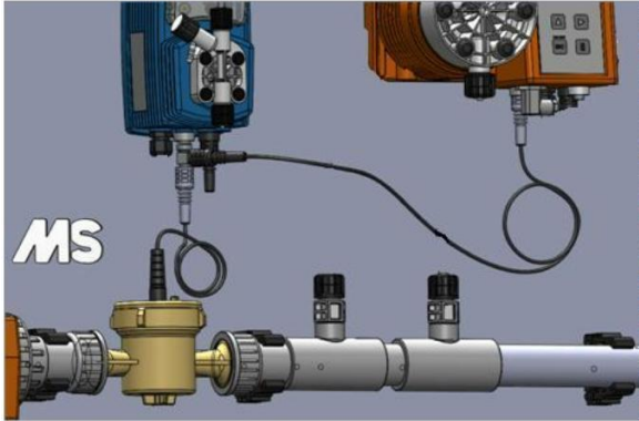
III. 5 : Connexion du débitmètre
