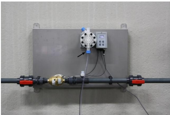
Abbildung 3: Saugschlauch anschließen
