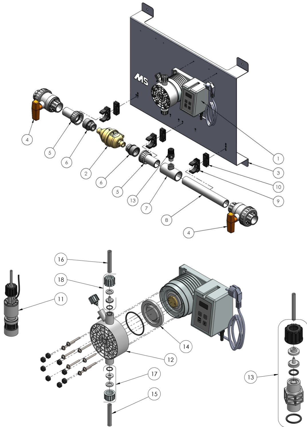
Abb. 1.1 Explosionszeichnung
