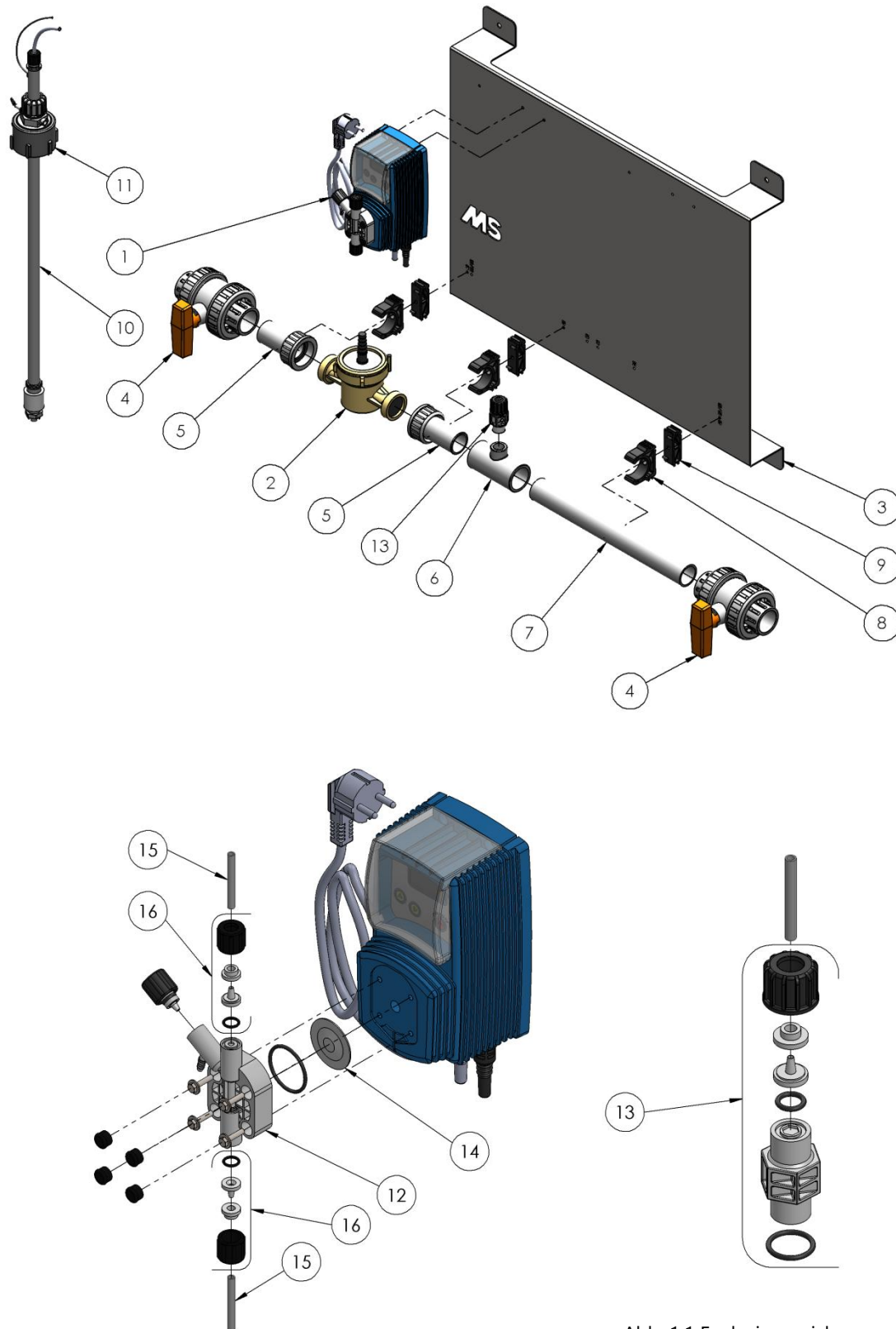
Abb. 1.1 Explosionszeichnung
