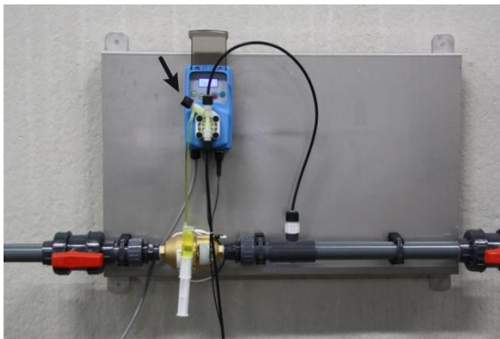
Abbildung 7: Pumpe entlüften
