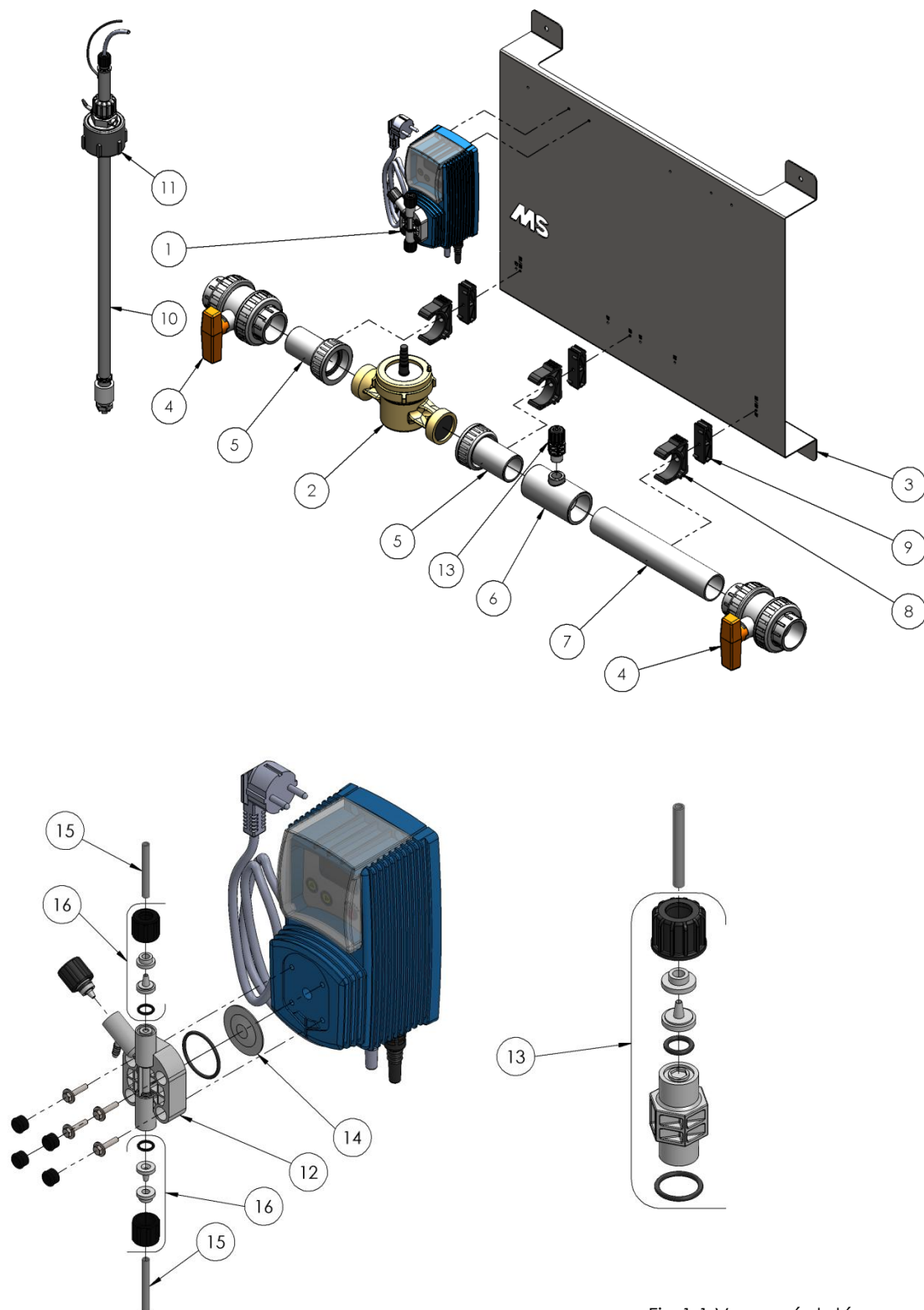
Fig 1.1 Vue en éclaté
