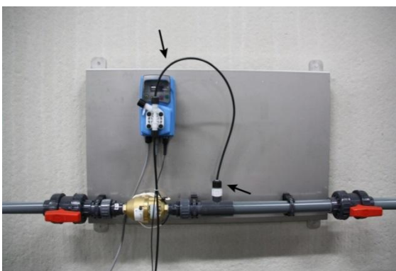
III. 4: Raccorder le tuyau de sortie
