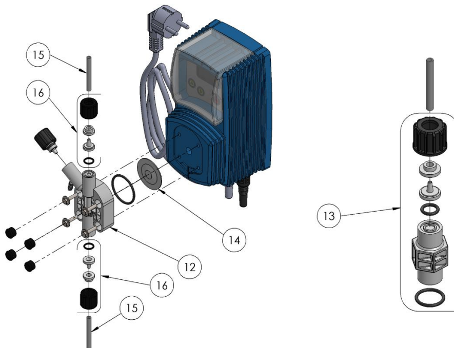
Fig 1.1 Vue en éclaté
