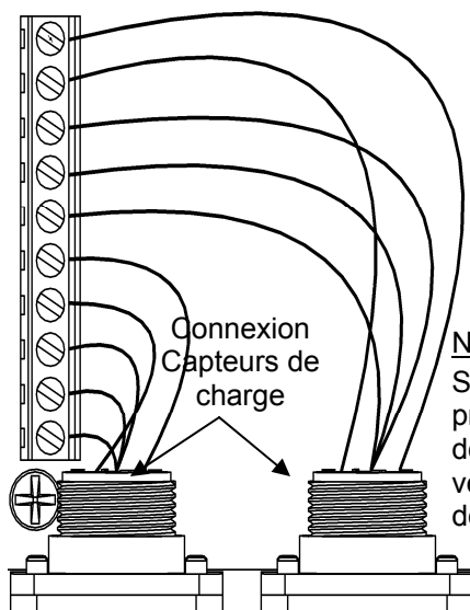
Diagramme Connexion des conducteurs
