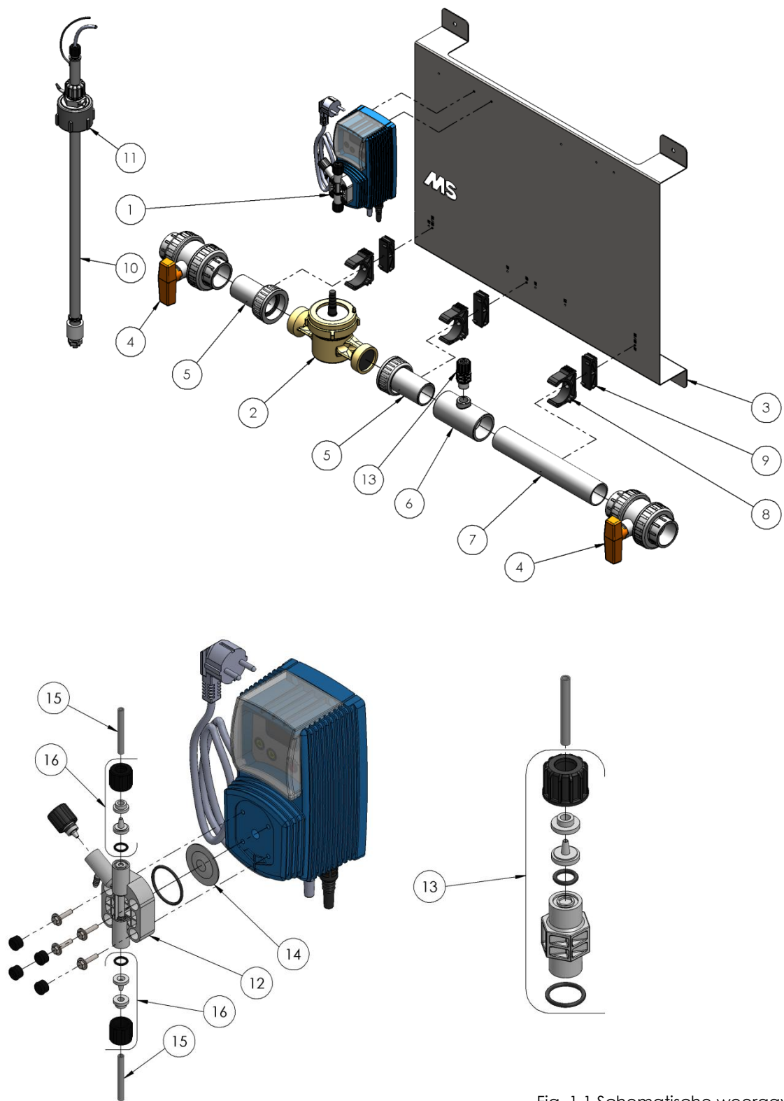
Fig. 1.1 Schematische weergave
