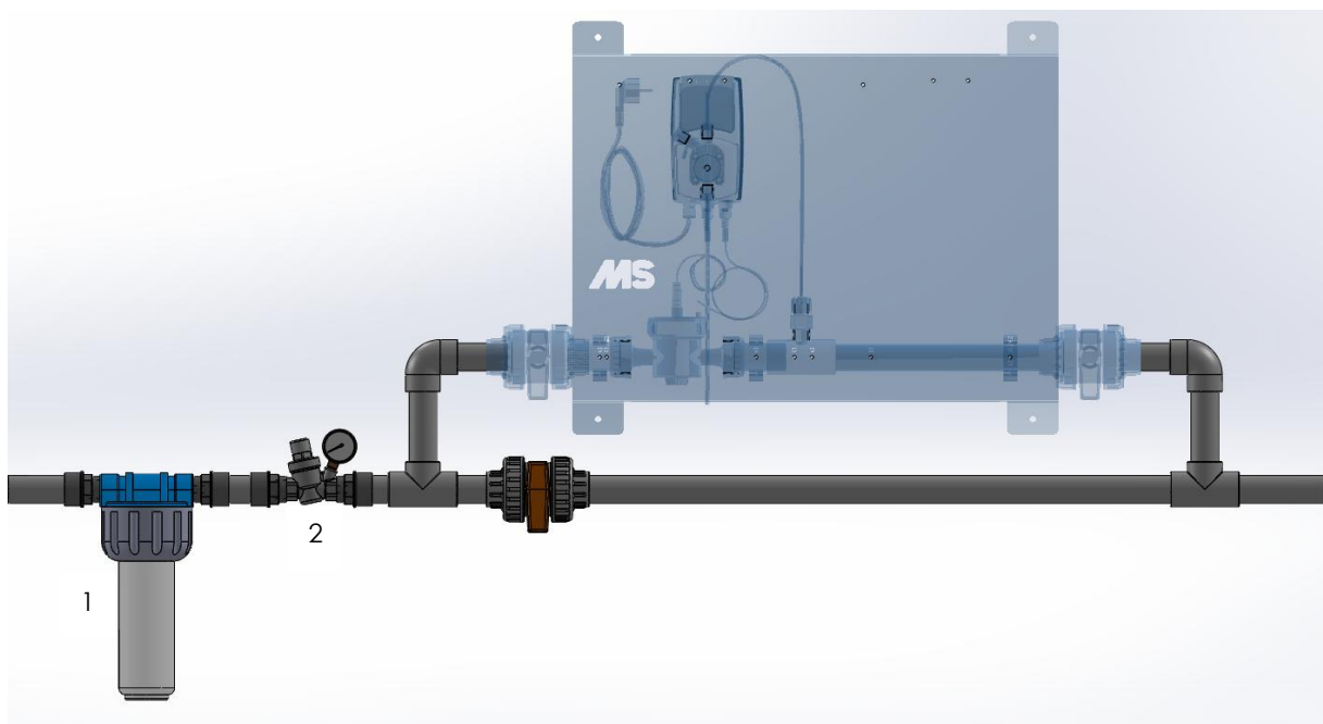
Fig. 2.1 Schematische weergave
