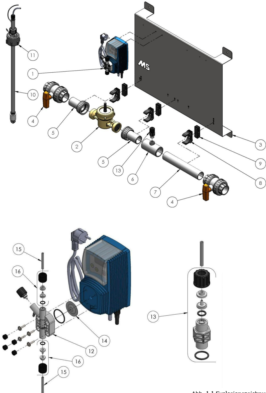
Abb. 1.1 Explosionszeichnung
