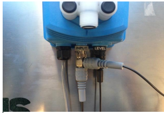
Imagen 2: Conexión de la protección contra el funcionamiento en seco y el contador de agua
