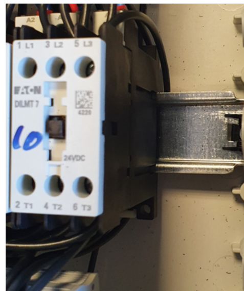
Figuur 4: relais in der Schiene.
